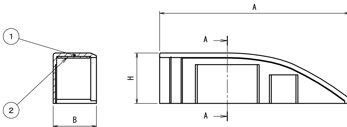
A-A断面図
